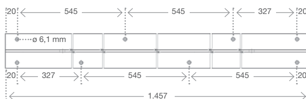
Lochbild der Bodenschiene B
