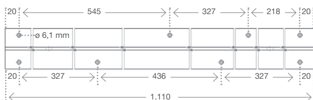
Lochbild der Bodenschiene A
